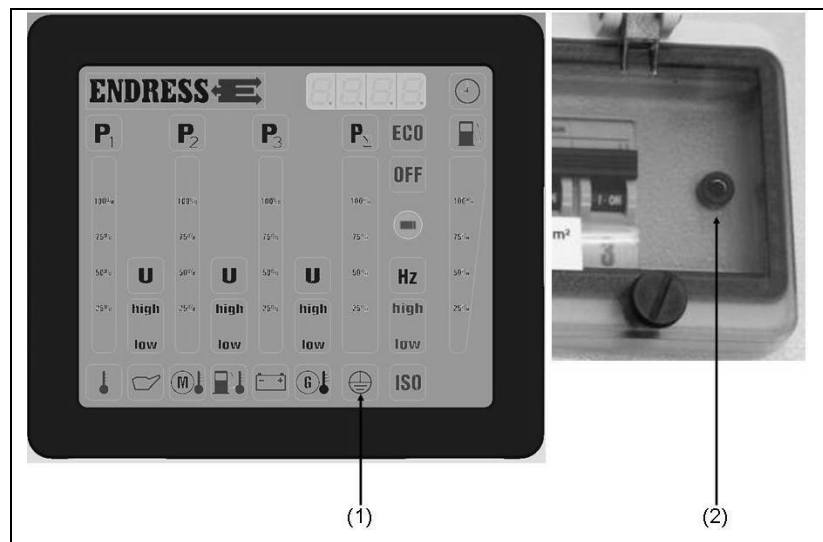
Ilustracja 4-4: Sprawdzanie przewodu ochronnego
