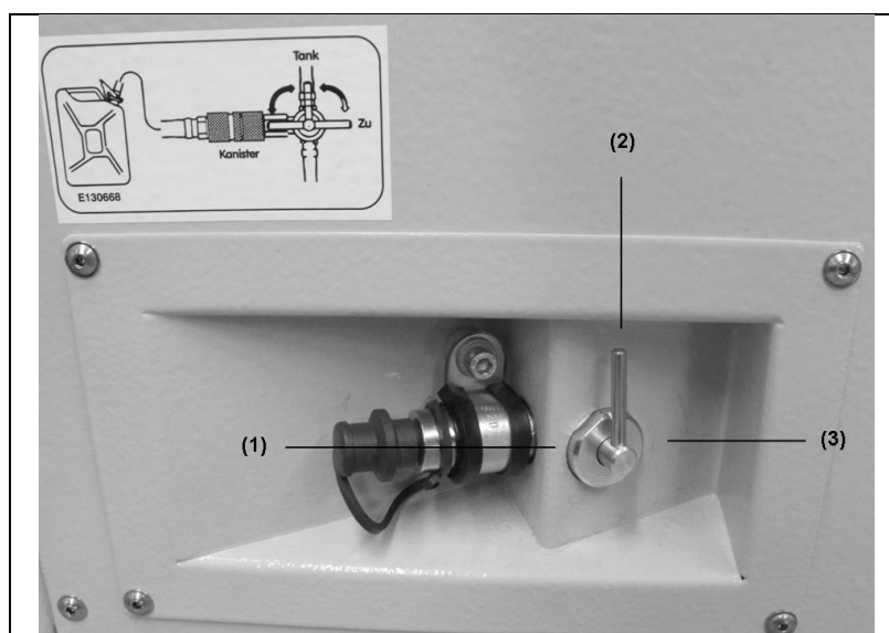
Ilustracja 5-10: 3-drożny zawór paliwa
