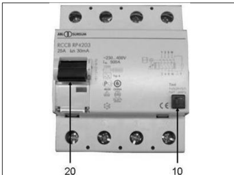
Ilustracja 5-1: Bezpiecznik różnicowo prądowy
