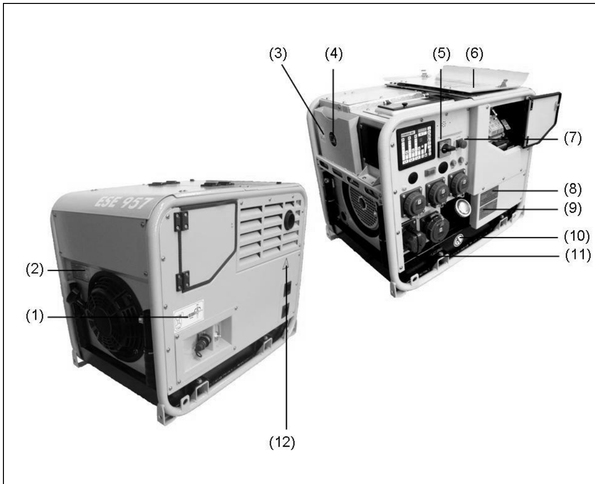
Ilustracja 2-1: Oznaczenia na agregacie prądotwórczym
