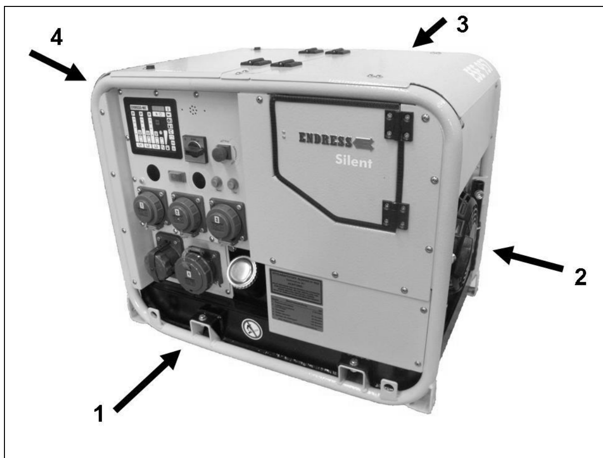
Ilustracja 3-1: Widok ogólny agregatu prądotwórczego
