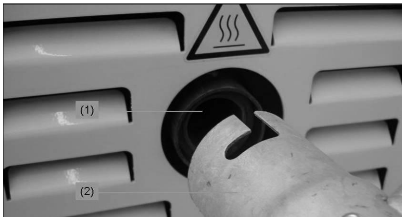
Ilustracja 5-11 Podłączanie węża do odprowadzania spalin
