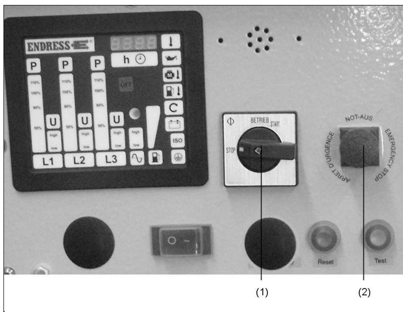
Ilustracja 4-2: Panel sterowania wersji standardowej
