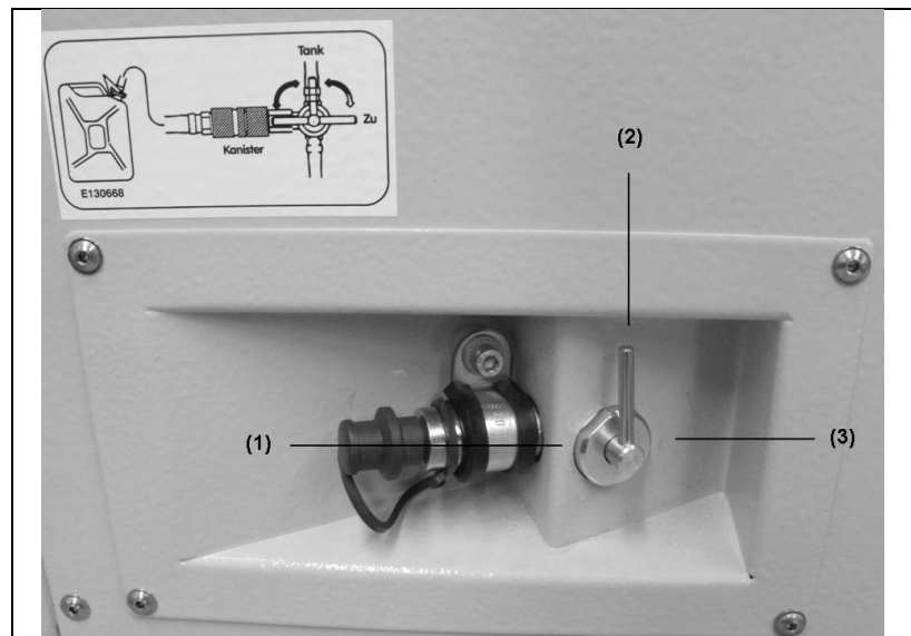
Abb. 5-11: 3 Wege Kraftstoffhahn
