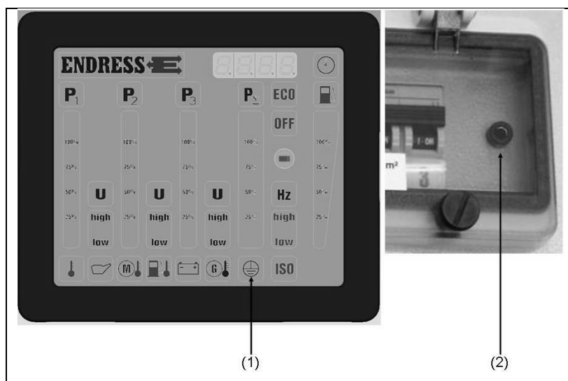
Abb. 4-4: Schutzleiter prüfen
