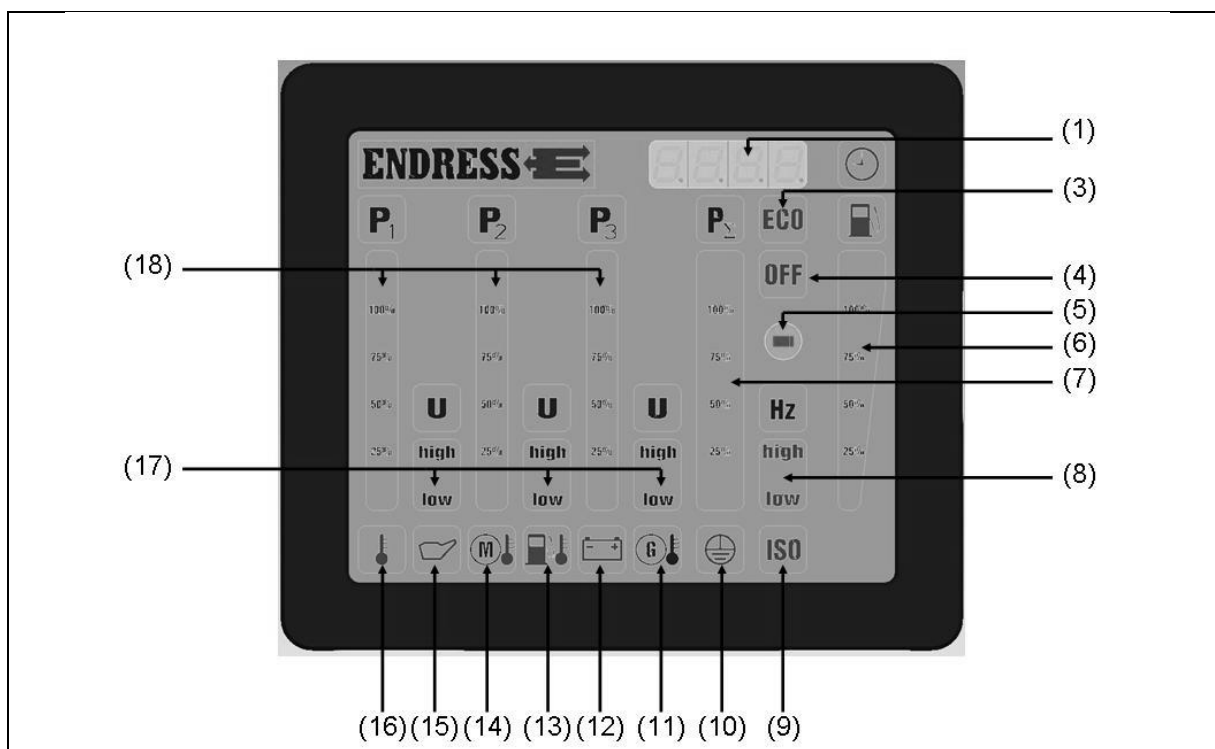
Abb. 4-5: Multifunktionsdisplay
