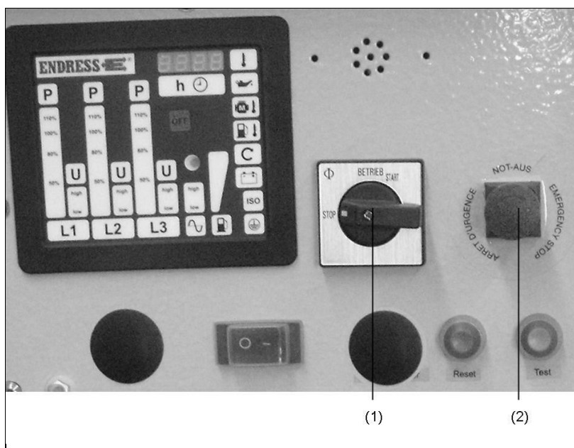
Abb. 4-2: Bedienpaneel Standardausführung
