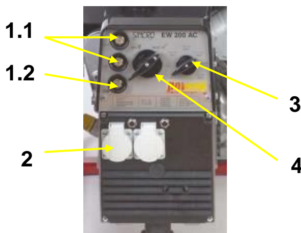
Рис. 4.3: Подключение потребителей
