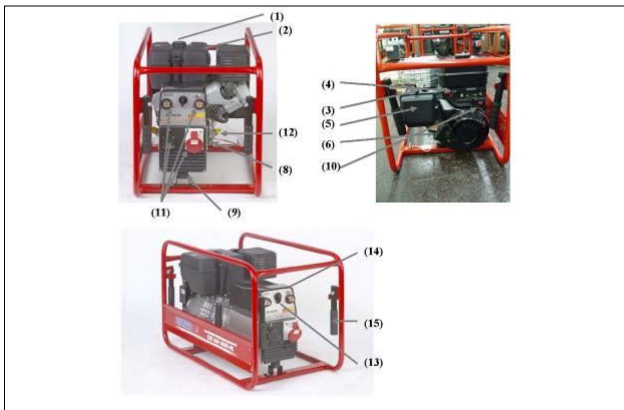
Рис. 3.1. Элементы электростанции
