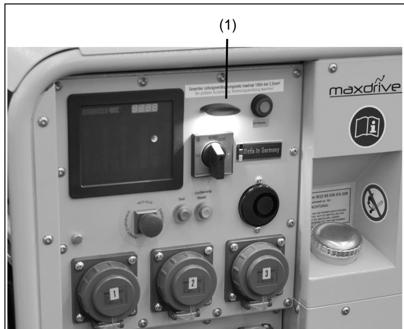
Abb. 4-3: Bedienpaneel mit Option Bedienfeldbeleuchtung
