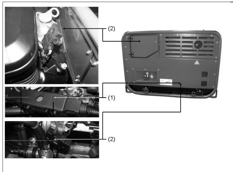
Abb. 6-4: Sicherung tauschen
