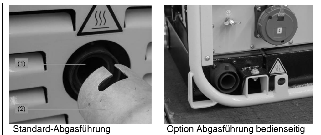
Abb. 5-13 Abgasschlauch anschließen
