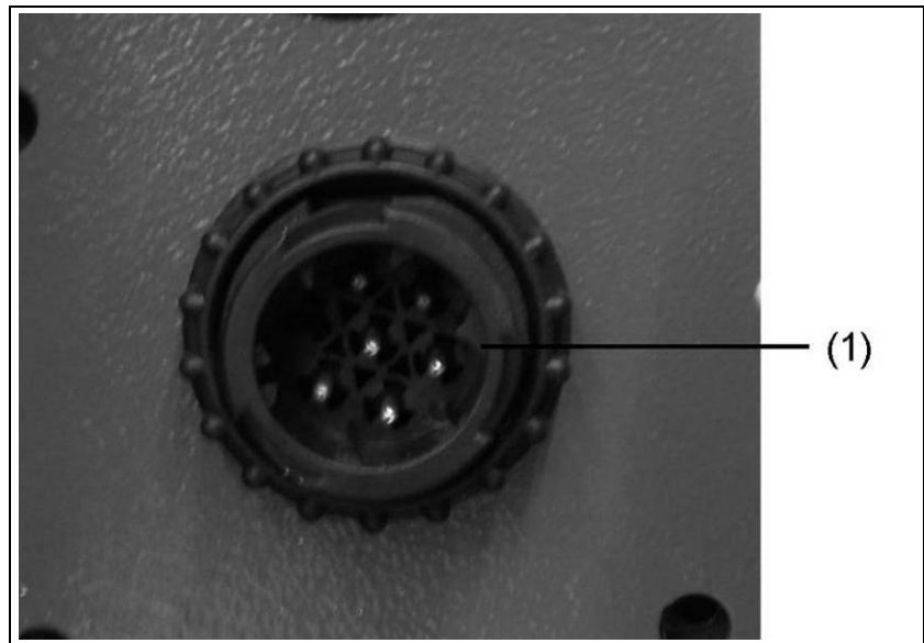
Abb. 5-6: Fernstarteinrichtung mit CAN-Steckdose
