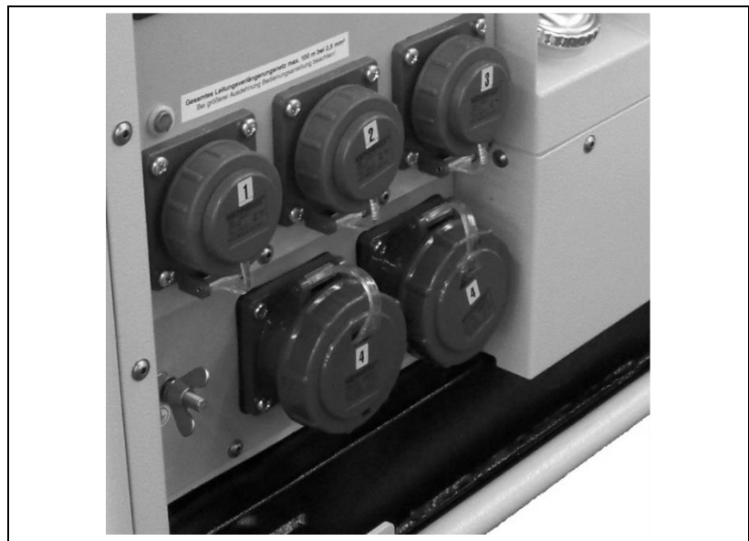
Abb. 4-4: Verbraucher anschließen
