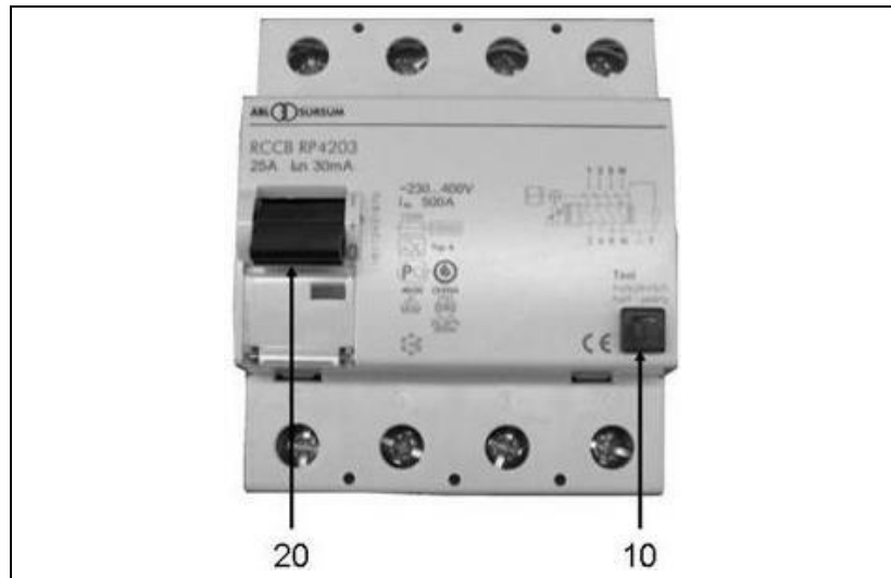
Abb. 5-1: FI-Schutzschalter
